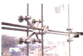
点支式玻璃幕墙“爪”型连接件
