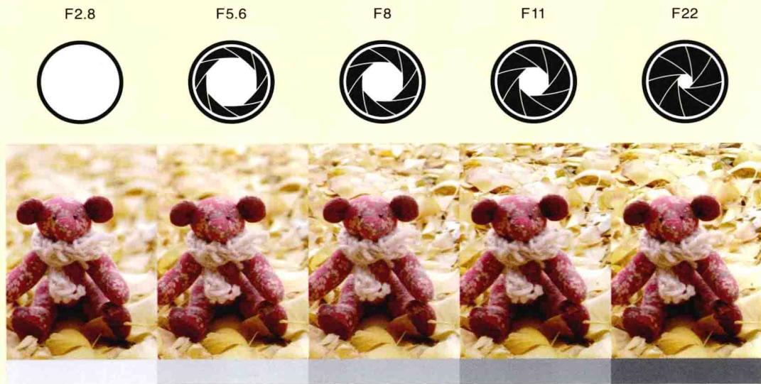
光圈值与光圈大小、背景的虚化程度及亮度的关系一览表
