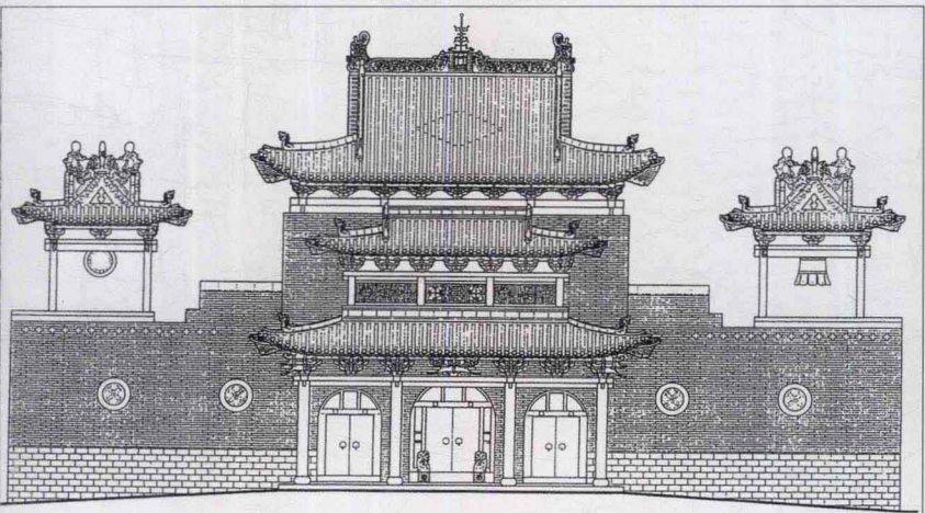
山西临县碛口镇黑龙庙正面图
