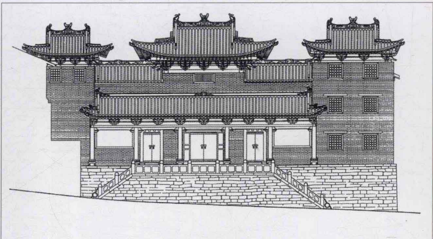
山西阳城郭峪村汤帝庙正面图
