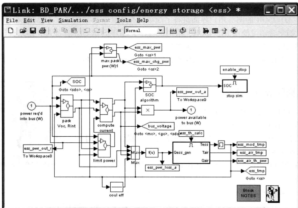
图 1-4 电池的电化学模型
