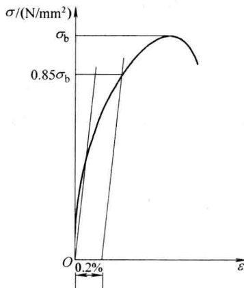
图 1-3 无明显流幅的钢筋的拉伸应力-应变曲线
