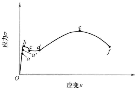
图 1-1 有明显流幅的钢筋的 拉伸应力-应变曲线
