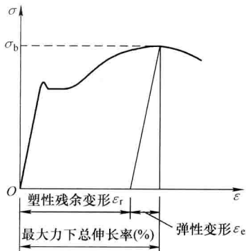
图 1-5 钢筋最大力下的总伸长率
