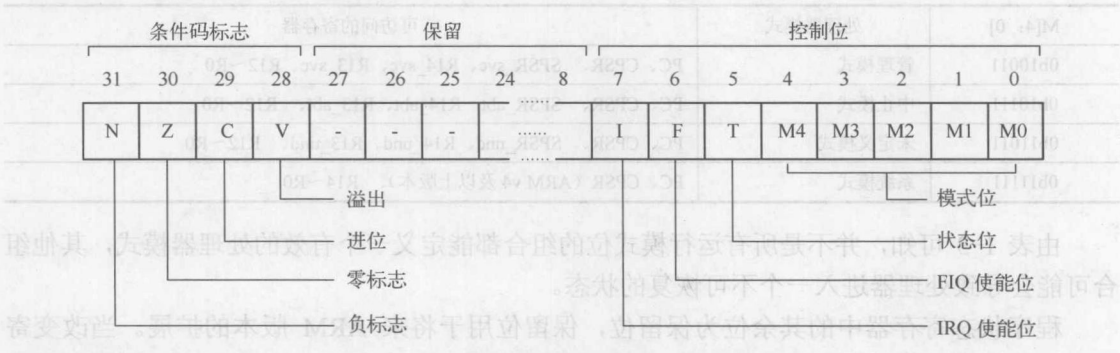
图 1-7 程序状态寄存器
