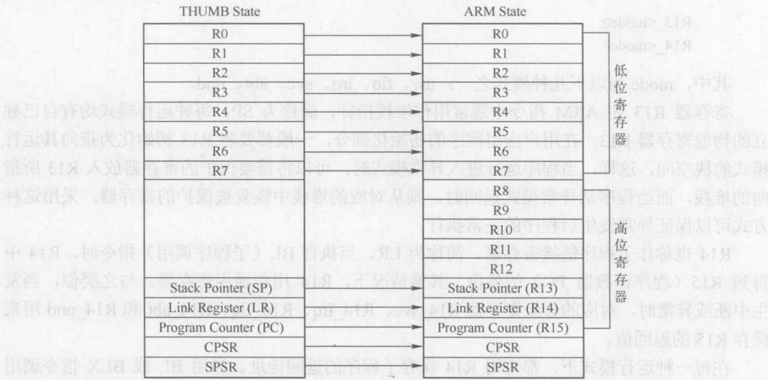
图 1-6 Thumb 状态寄存器映射到 ARM 状态寄存器
