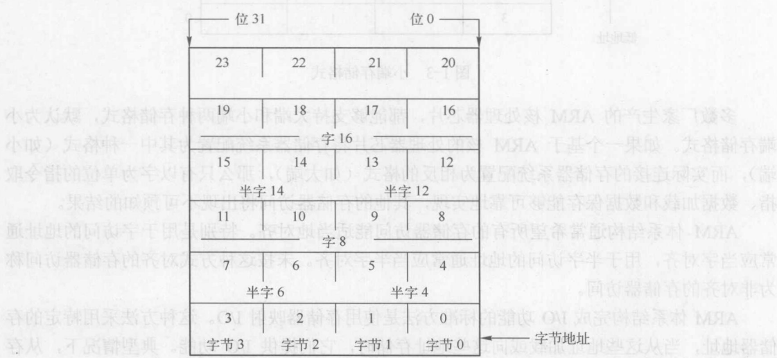
图 1-1 ARM 数据类型存储图
