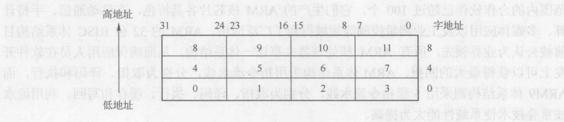
图 1-2 大端存储格式
