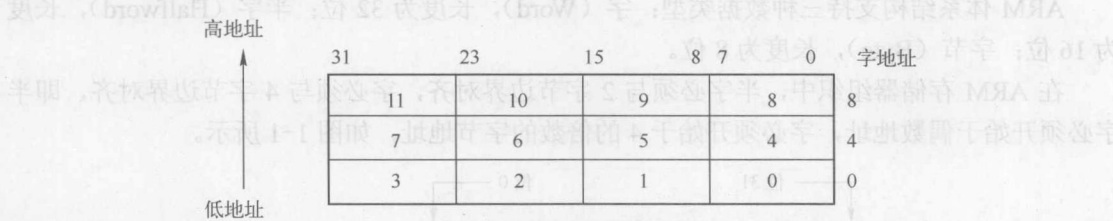
图 1-3 小端存储格式
