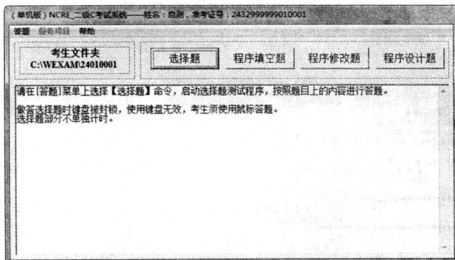
图 1.5 答题菜单
