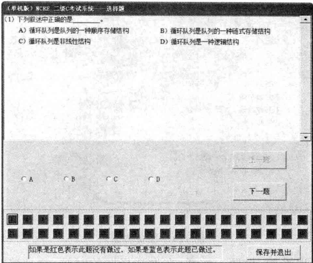
图 1.6 选择题
