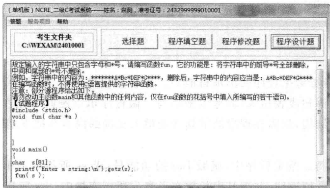
图 1.9 程序设计题
