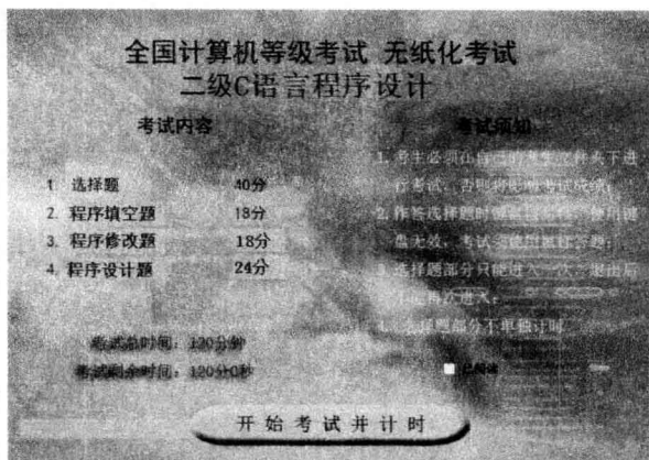
图 1.4 准备答题
