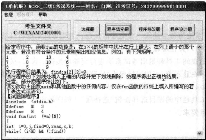
图 1.7 程序填空题
