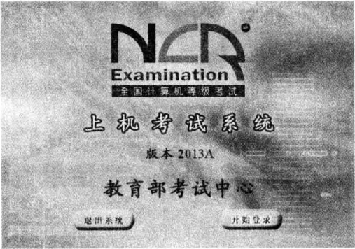
图 1.1 登录界面
