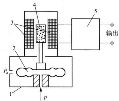
1—壳体；2—膜盒；3—电感线圈；4—磁芯；5—转换电路
