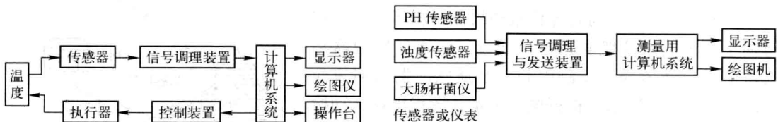
图 1.7 电炉温度自动检测与控制系统组成框图
