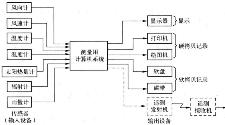
图 1.1 气象参数自动检测系统示意图
