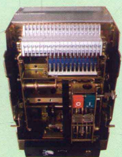
DW50-1000 抽框架
