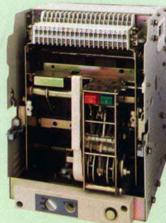
DW60-1250 抽框架
