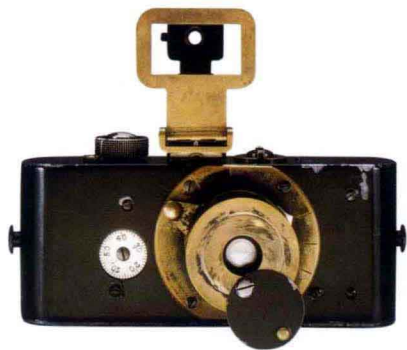
图2 Ur-Leica
