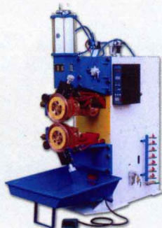
FN1-160-1 缝焊机
