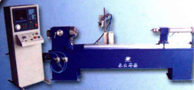
HF数控环缝焊机
