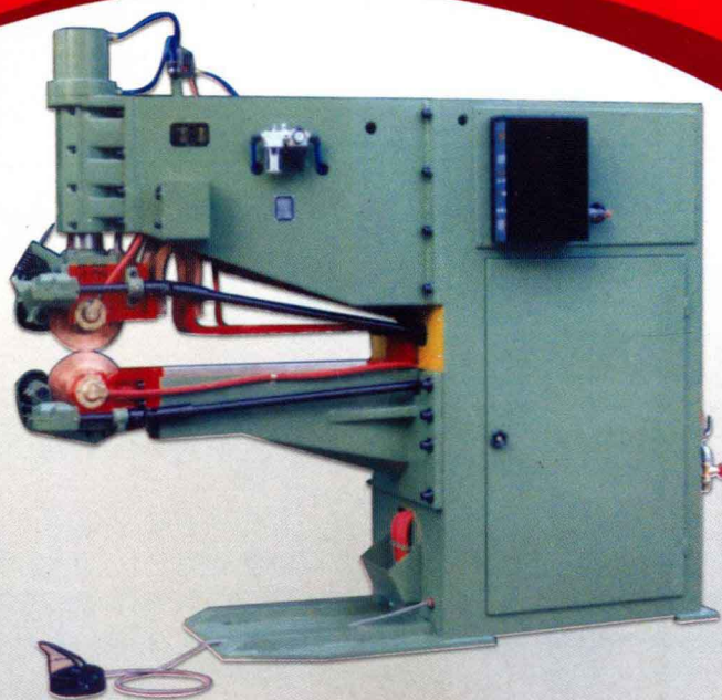
FN1-150-5缝焊机
