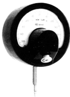
图 2.4 扭簧比较仪
