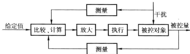
图1-9 复合控制系统框图
