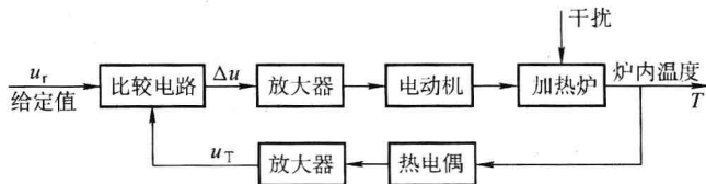
图 1-2 加热炉温度控制系统框图
