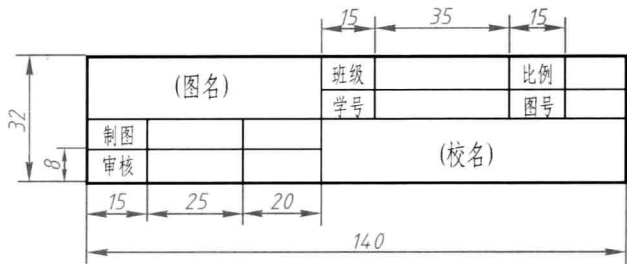
图 1-7 标题栏格式(制图作业中使用)
