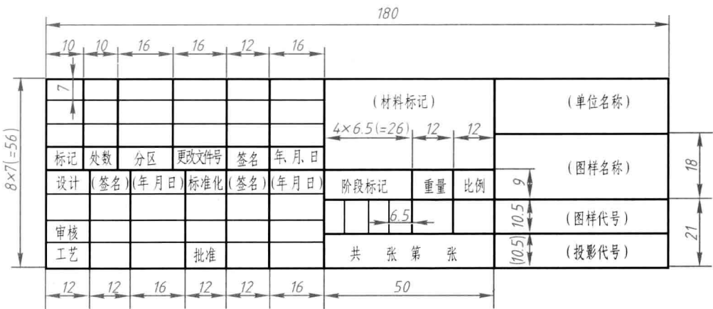
图 1-6 标题栏格式举例
