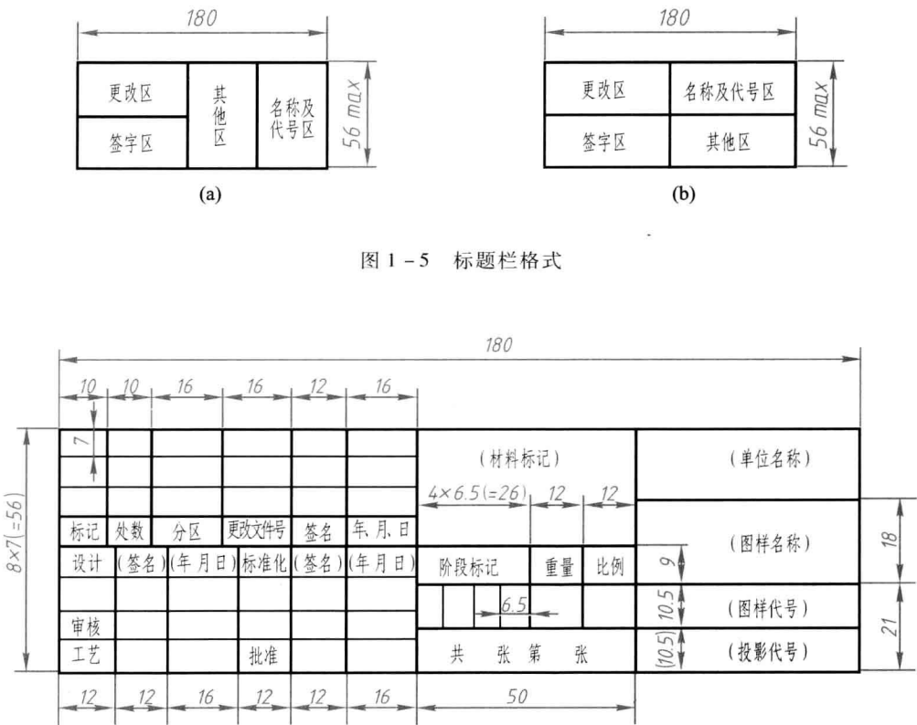
图 1-6 标题栏格式举例
