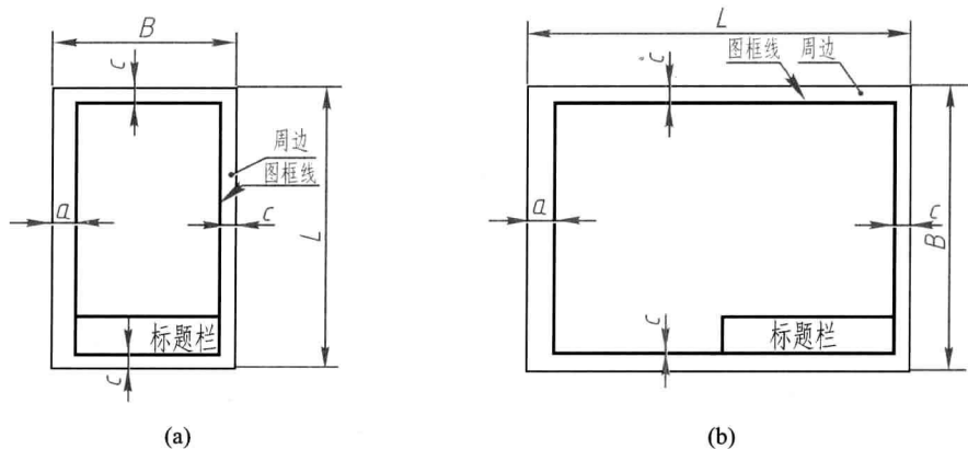
图 1-2 图框格式
