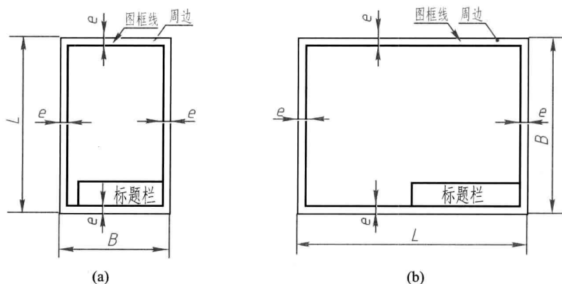
图 1-3 图框格式
