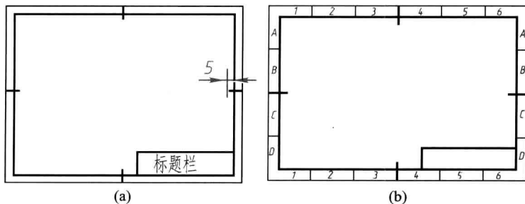
图 1-4 图幅的对中符号与分区
