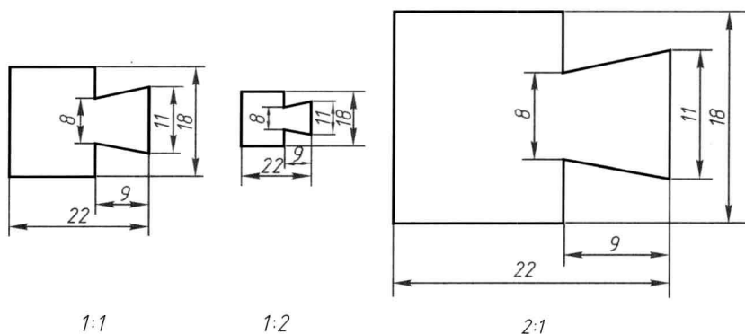
图 1-8 图形比例与尺寸标注
