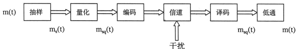
图 1-3-3 脉冲编码调制原理
