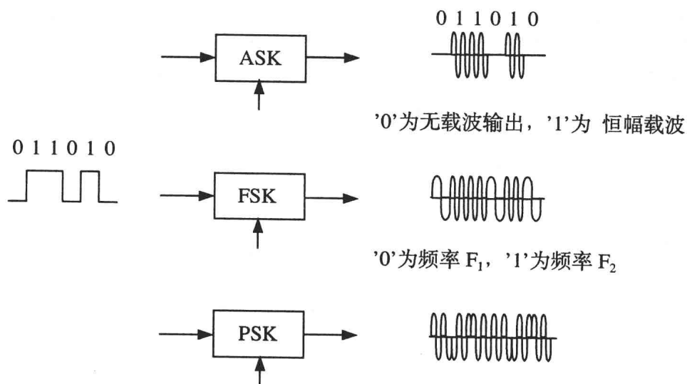
图 1-3-2 基本的数字调制方式
