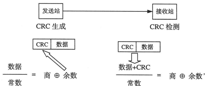
图 1-3-4 循环冗余校验的基本原理
