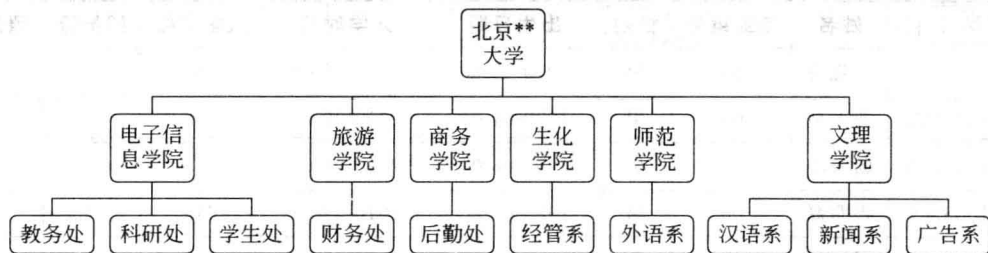
图 1-3 层次模型
