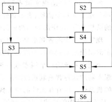
图 1-4 网状模型
