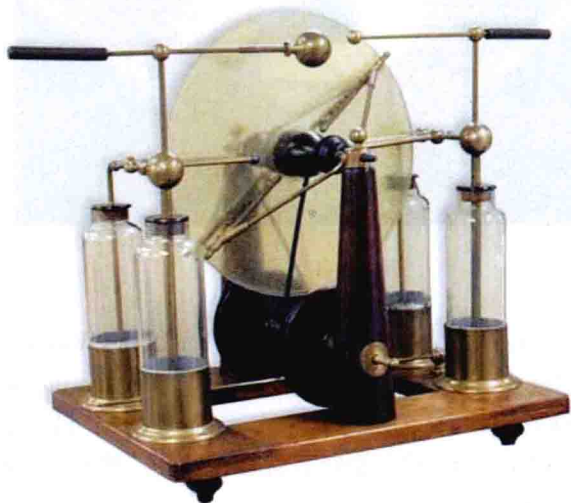
■ 图 1-3 带有莱顿瓶的摩擦起电机
