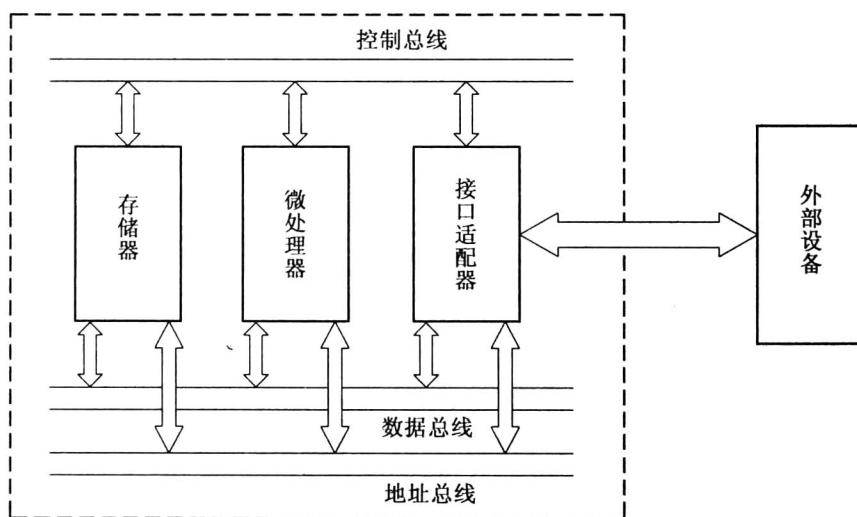
图 1-1 单片机的组成
