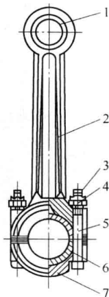
图 1-5 内燃机连杆
