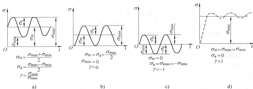
图 1-7 应力的循环种类
