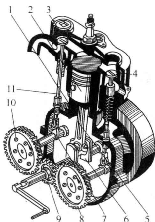
图 1-3 内燃机
