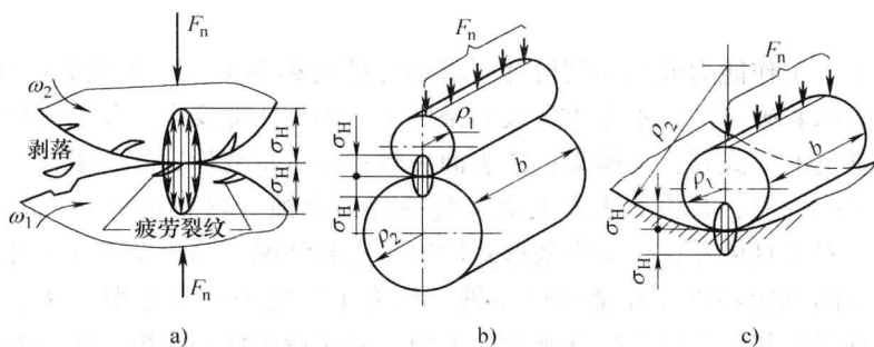
图 1-6 疲劳点触和接触应力计算模型
