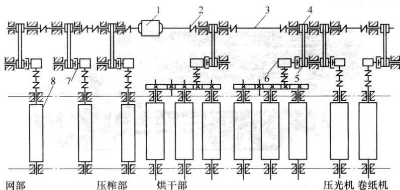
图 1-2 造纸机简图
