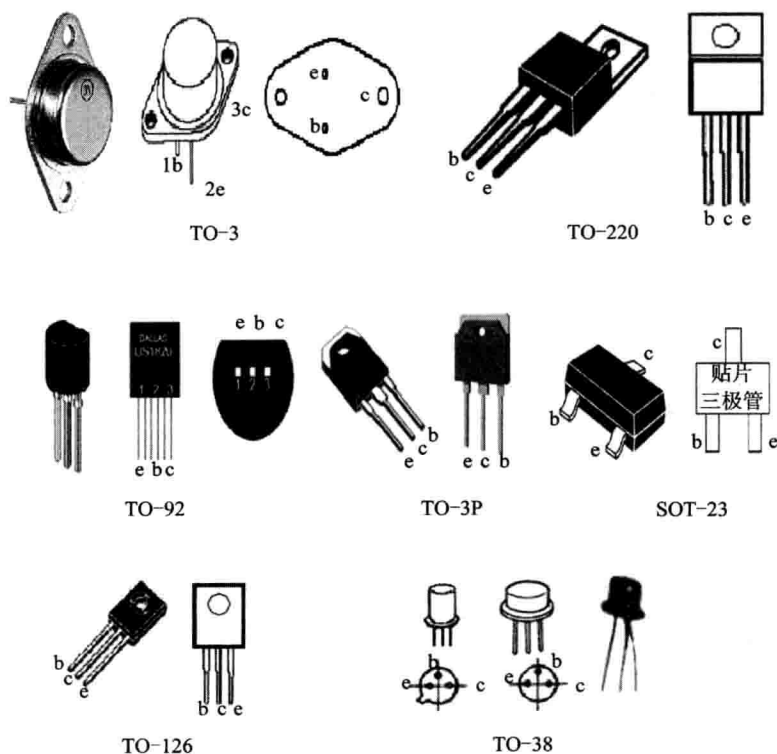
图 2.5 常见三极管的型号和引脚排列
