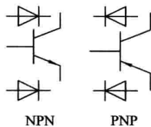
图 2.4 晶体三极管的等效结构
