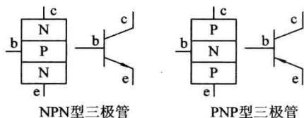
图 2.3 晶体三极管的结构及电路符号
