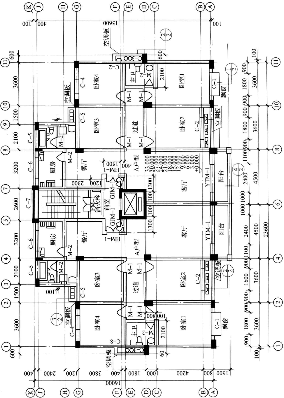
图 1.6.1-1 标准层平面图
