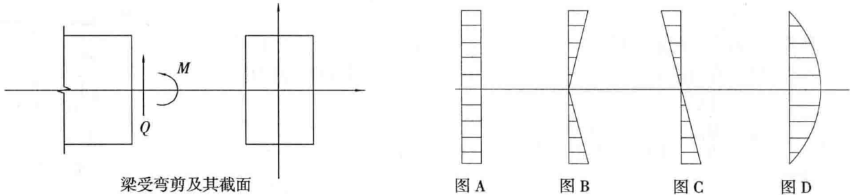
截面剪应力分布图
