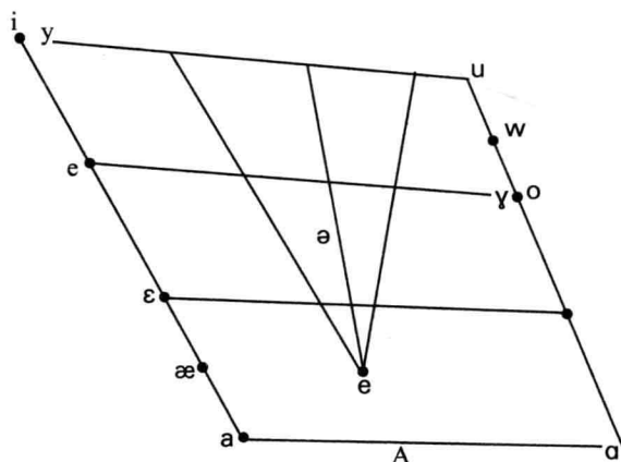
图2 舌面元音图
