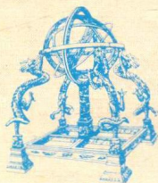
浑仪 中国铜制天文仪器，公元1437年仿制，现陈列于南京紫金山天文台。
