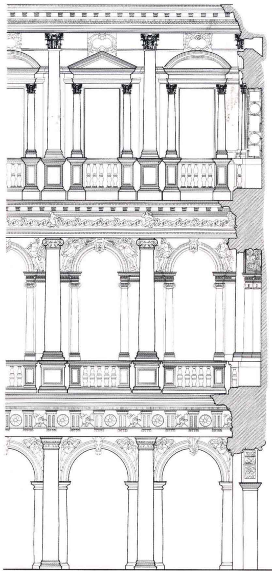
局部立面
