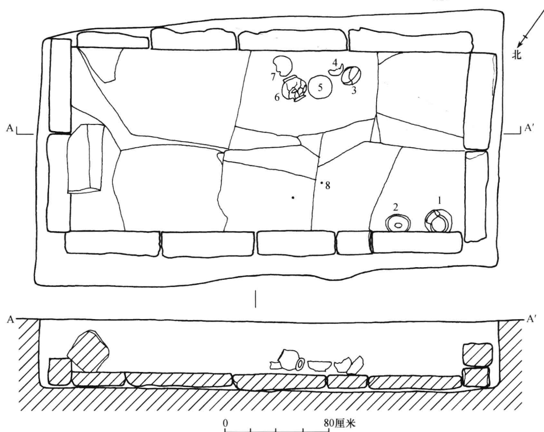
图三九八 2005FRWBM2平、剖面图
