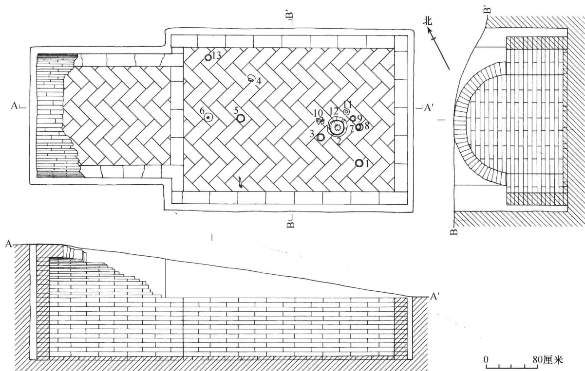
图四〇六 2005FRWBM5平、剖面图
