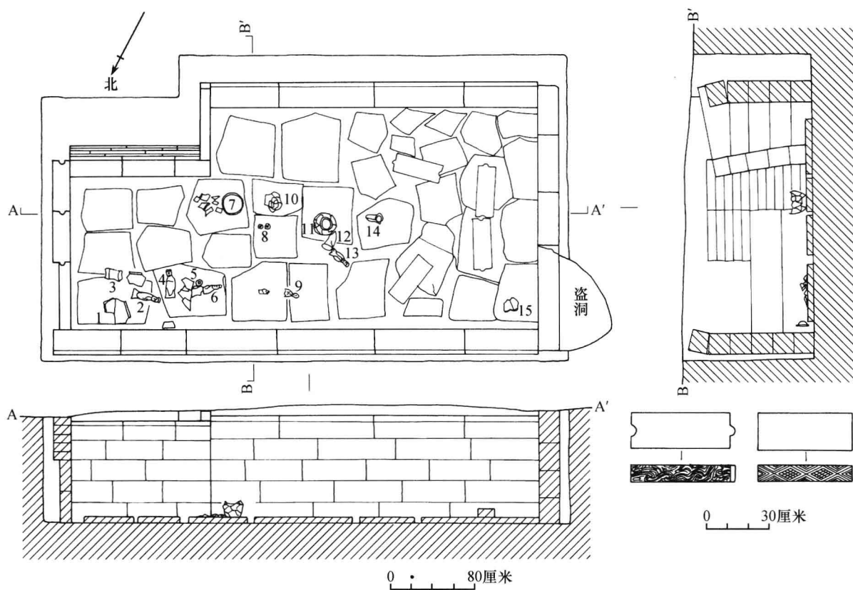
图四〇〇 2005FRWBM3平、剖面图
