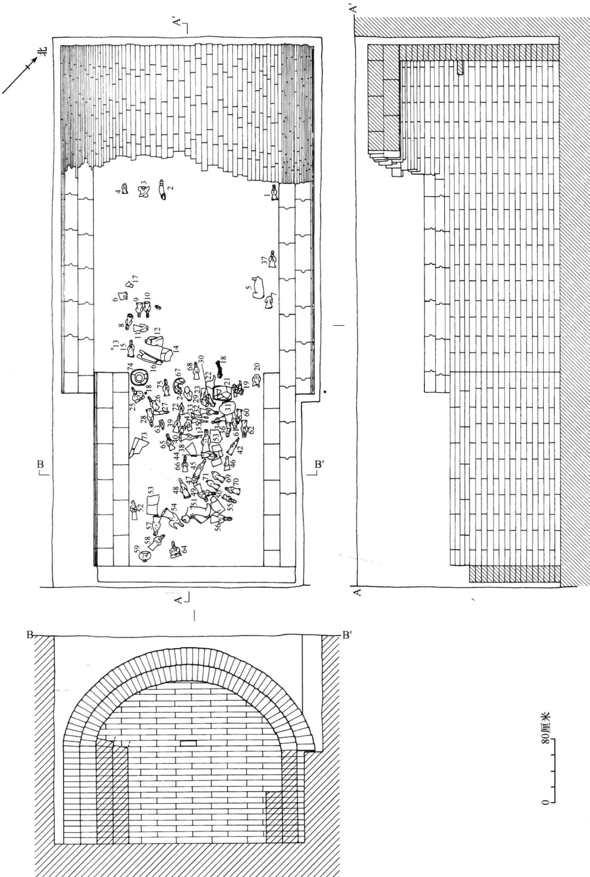
图四〇九 2005FRWBM6平、剖面图
