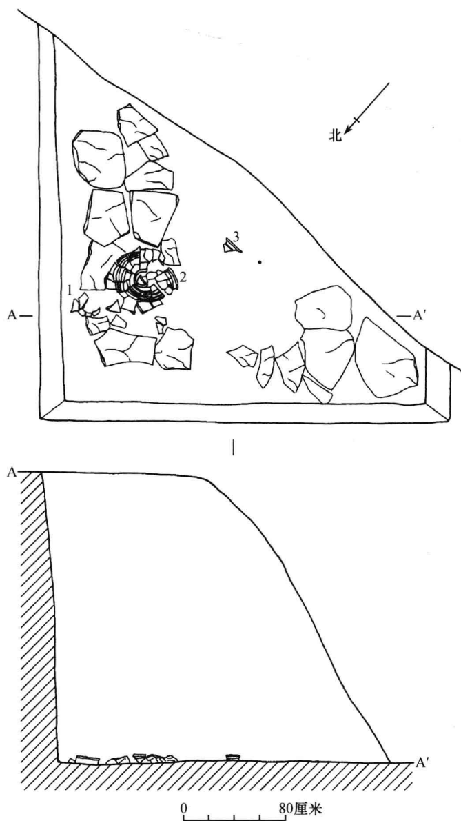
图四〇四 2005FRWBM4平、剖面图
