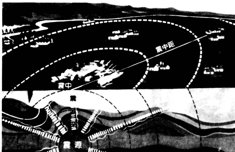
图 1.1 地震示意图
