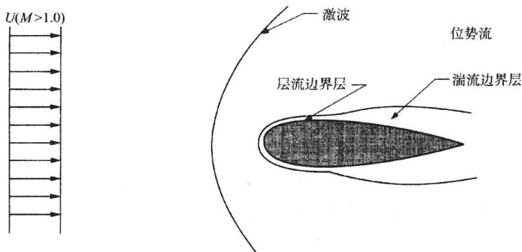
图 1-7 超声速绕流
