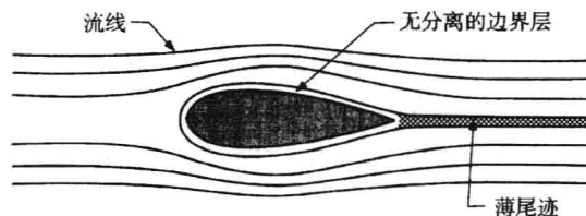
图 1-5 绕流线型物体的流动.尾缘缓慢地变尖,防止了边界层的分离
