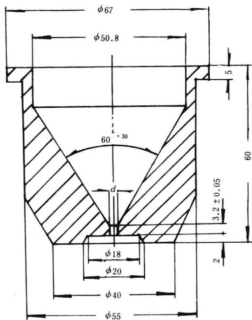
图 1 标准漏斗
