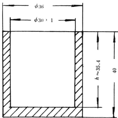
图 2 圆柱杯
