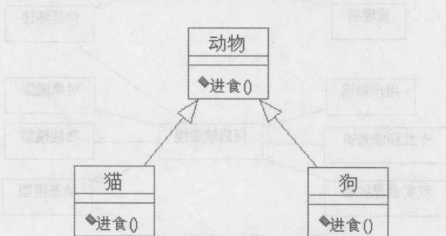
图 1-2 图形多态性示例
