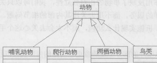
图 1-1 动物类继承结构示例
