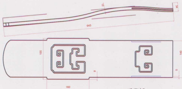
03 后背板
