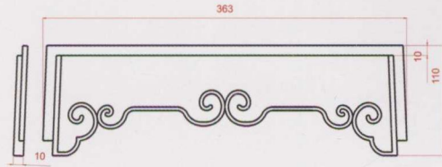
06牙板
