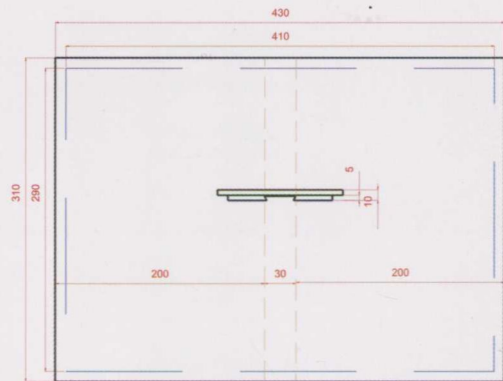
5.4 座板
