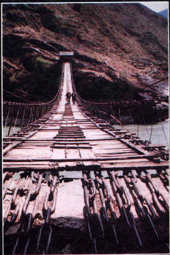
长江第一桥金龙桥
