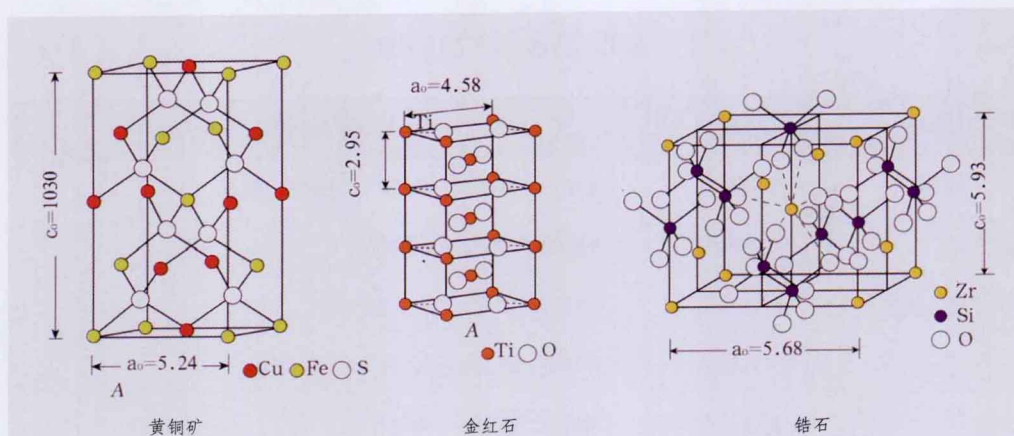
几种矿物晶体内部质点的排列方式 (数字表示质点排列的间距, 以 A=10^{-10} 米为单位)
