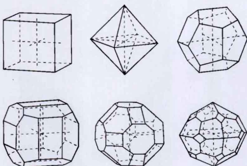
等轴晶系常见的晶体
