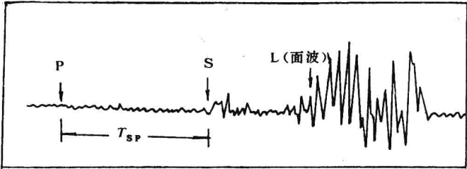
图 1-4 地震波记录图
