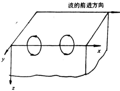
图 1-3 瑞雷波表面质点运动轨迹
