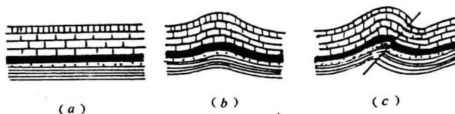
图 1-1 构造变动形成地震示意图
