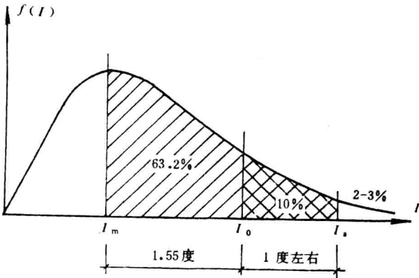
图 1-6 三种烈度的超越概率示意图
