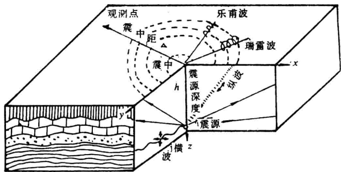
图 1-2 地震波传播示意图
