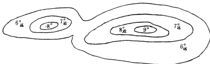
图 1-5 设计近震和远震的规范划分法
