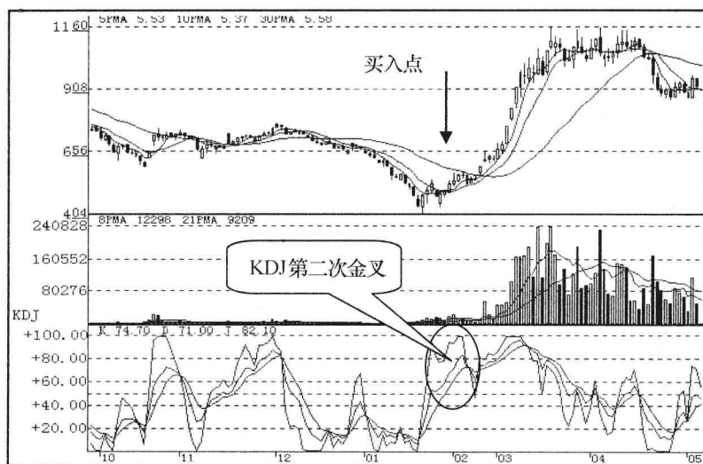
图 2—A KDJ、MA 指标走势图
