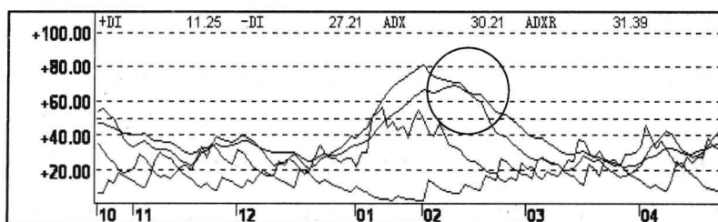
图 3—B DMI 指标走势图
