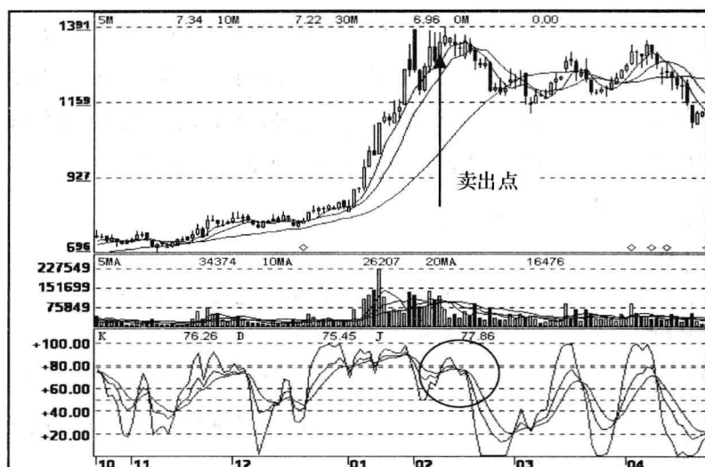
图 3—A KDJ、MA 指标走势图
