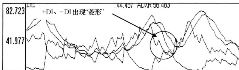
图 2—B DMI 指标走势图
