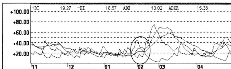
图 1—B DMI 指标走势图
