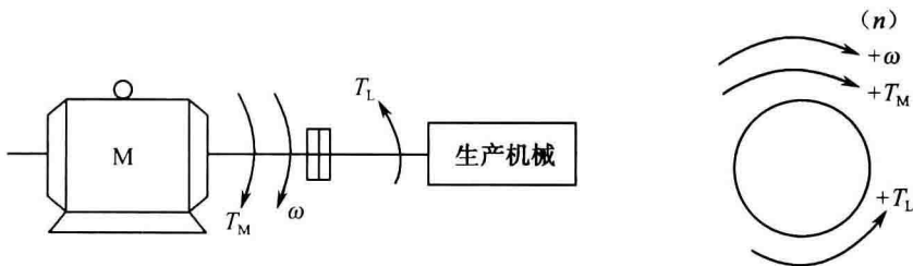
图 0-2 单轴机电传动系统
