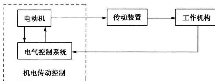
图 0-1 机电传动系统的组成框图
