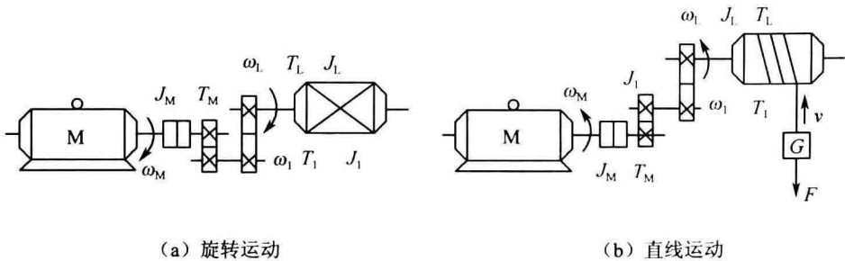
图 0-4 多轴机电传动系统
