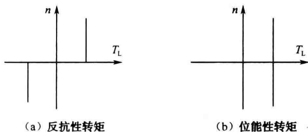
图 0-5 两种恒转矩型负载
