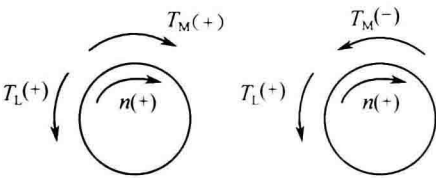
图 0-3 T_M 、 T_L 符号的约定
