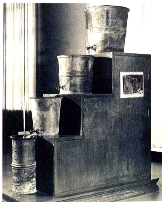
元朝製造的銅壺滴漏
