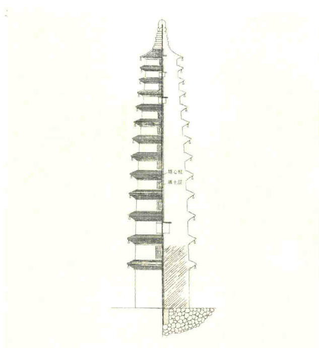
方塔结构推定示意图
