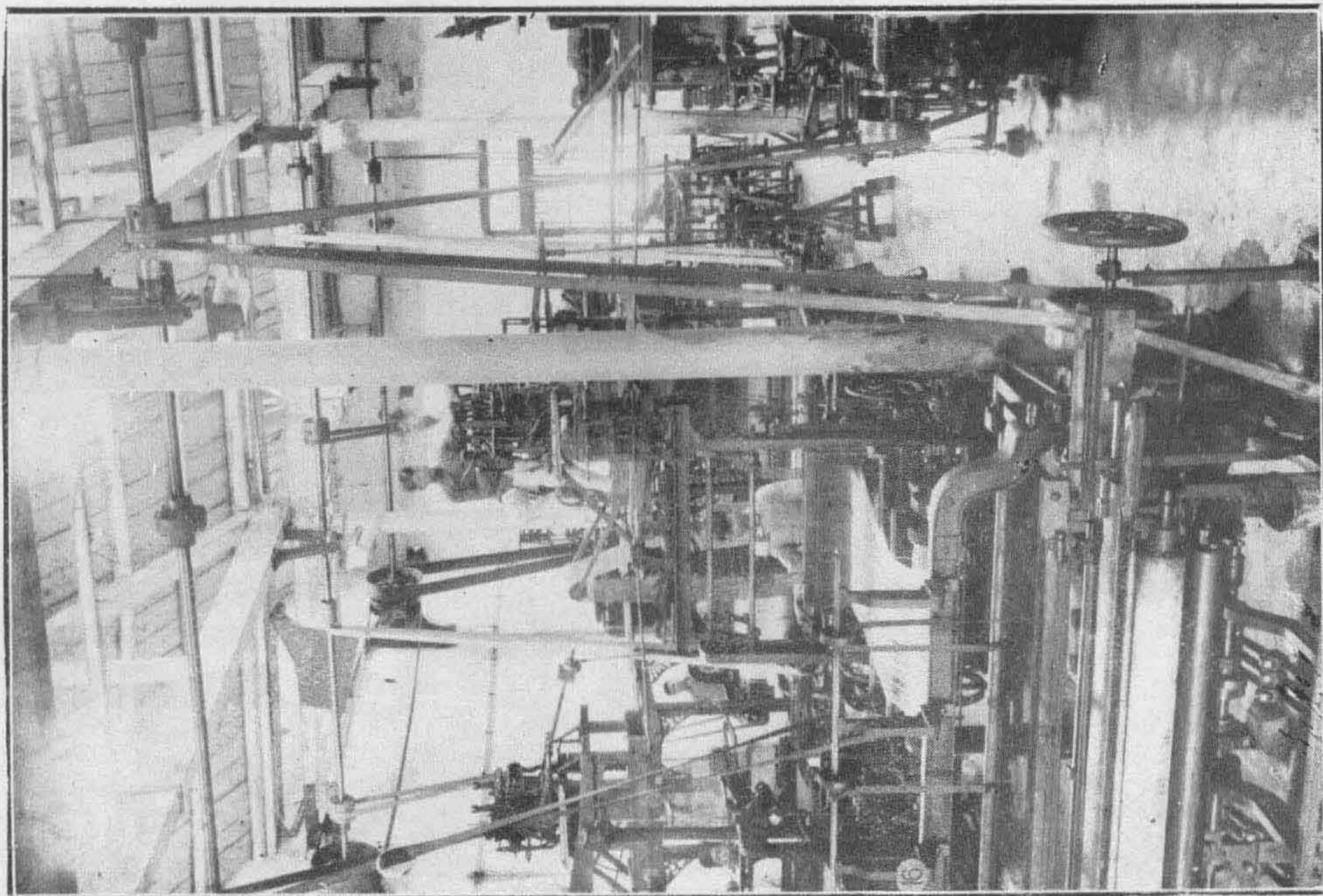
機織工場
