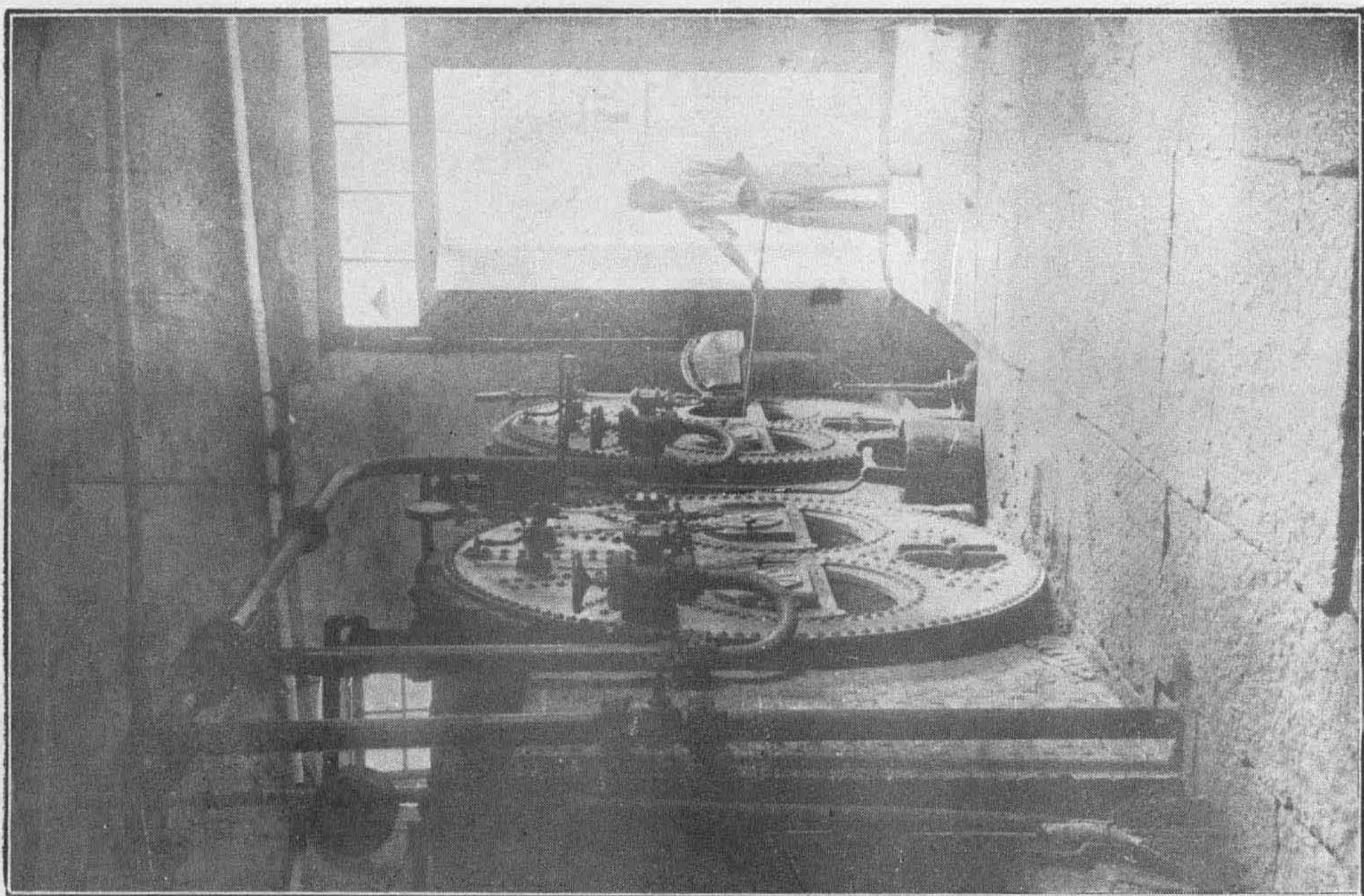
原動室
