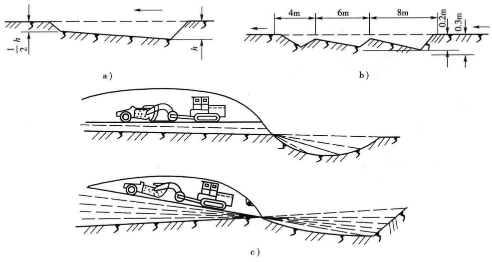
图 1-1-3 铲运机的工作
