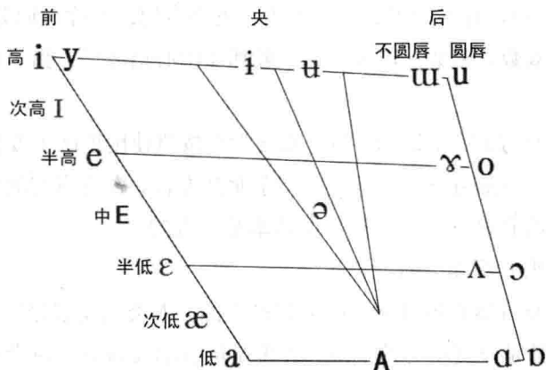
图 2 元音舌位图
