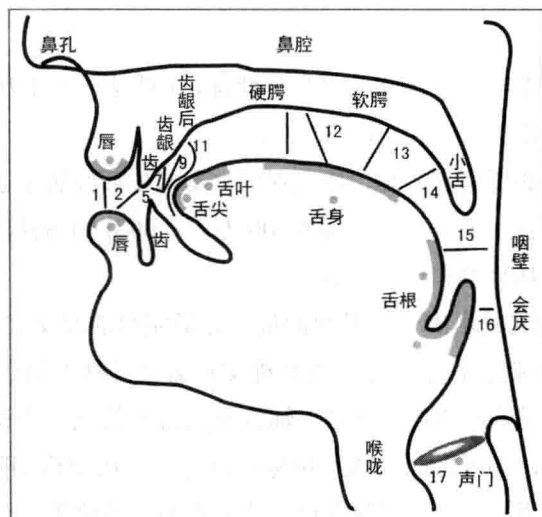
图 1 发音器官图
