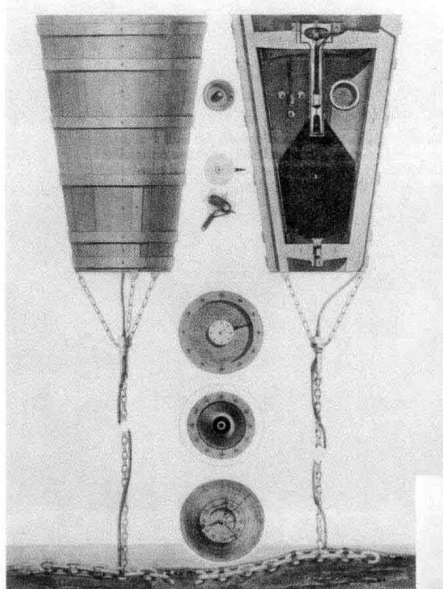
由诺贝尔父亲英马努艾尔设计的水雷
