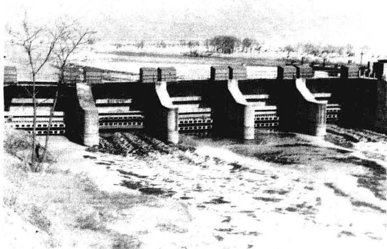
柏各庄农场东西灌区输水总干渠岩山渠首
