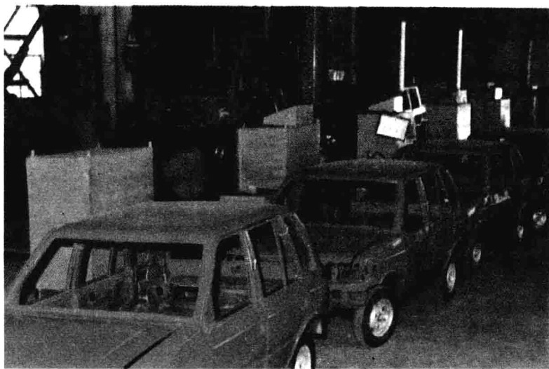
县汽车车身总厂“家庭”牌超微型轿车生产线
