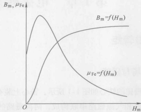
图 1-3 铁磁材料的磁化曲线 ( B_m = f(H_m) )
