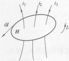
图 1-2 安培环路定律
