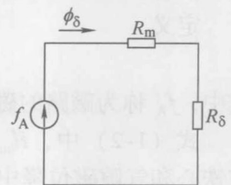
图 1-4 等效磁路图
