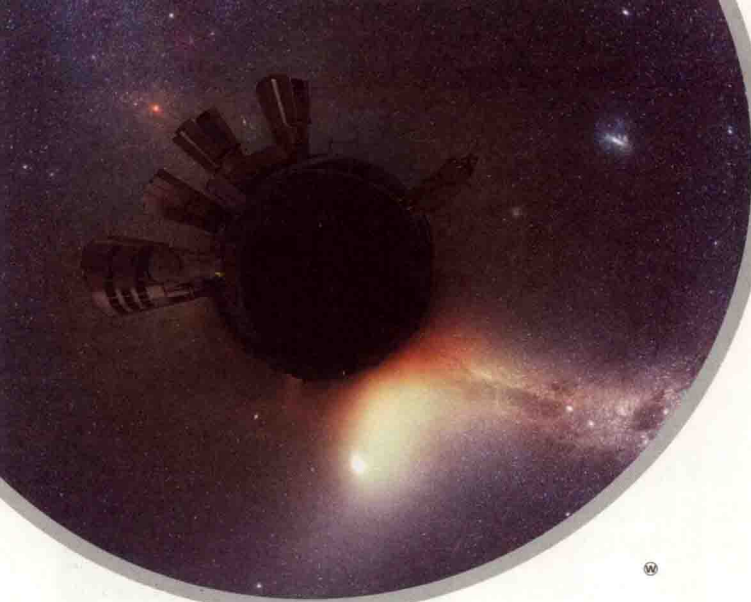
鱼镜头拍摄的帕拉纳尔天文台，天文学家关心的是大气层外的天体
