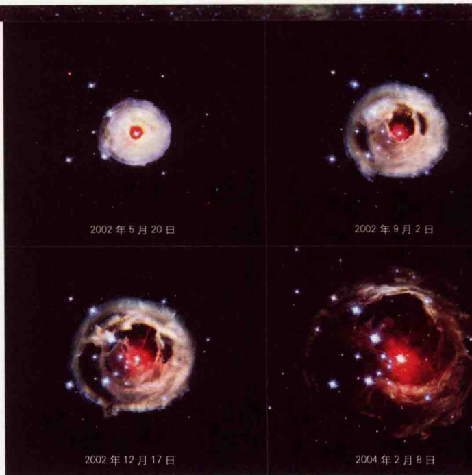
麒麟座 V838 也许是已知最大的恒星之一，2002 年曾发生剧烈的爆发
