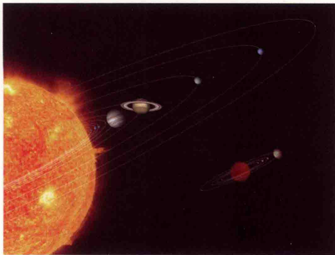
太阳系（左）和一颗红矮星的行星系统比较图
