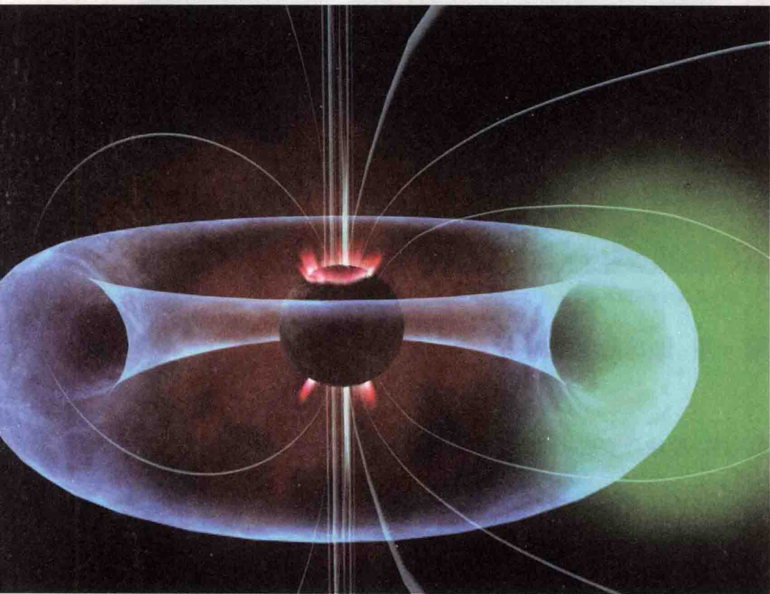
地球磁极的颠转确实存在着一个周期
