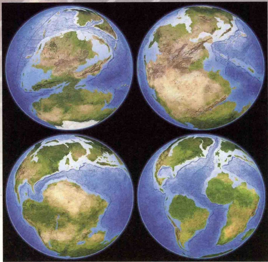
地球板块的演化与水密不可分
