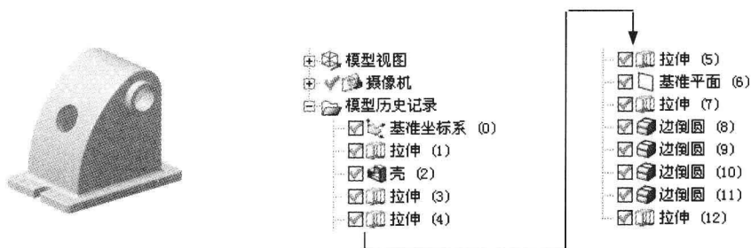
图 1.1 零件模型及模型树
