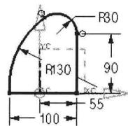
图 1.3 截面草图
