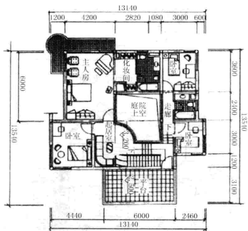
图4 二层平面图
