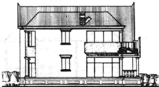
图8 西立面图
