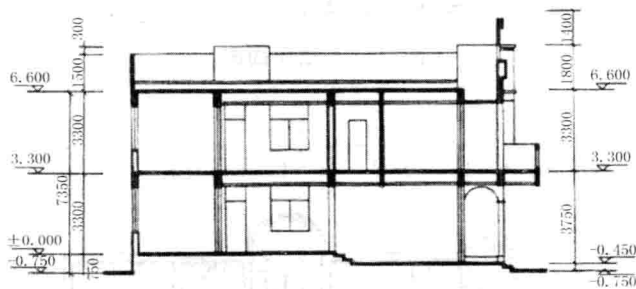
图 15 A-A 剖面图
