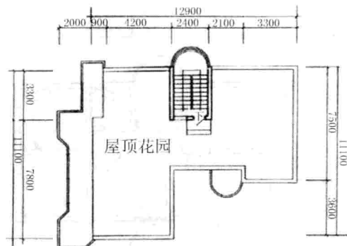
图 14 屋顶平面图
