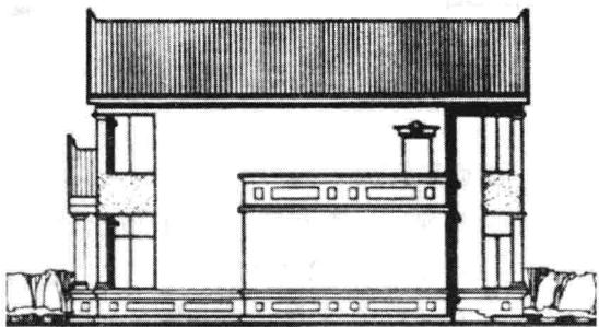
图9 东立面图
