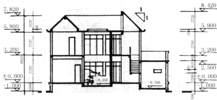
图 10 1-1 剖面图
