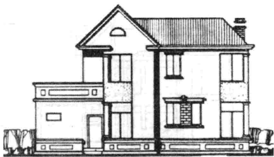
图7 北立面图
