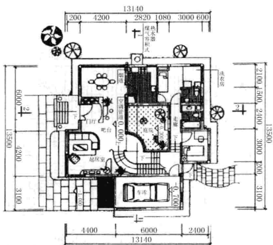
图3 一层平面图
