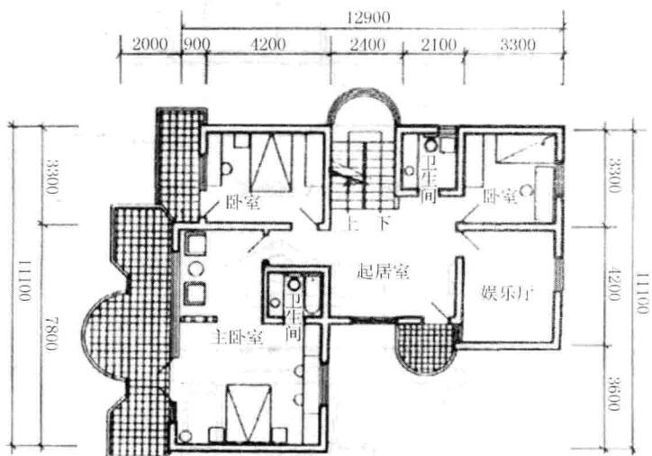
图 13 二层平面图
