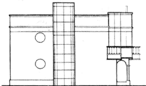
图 18 西立面图
