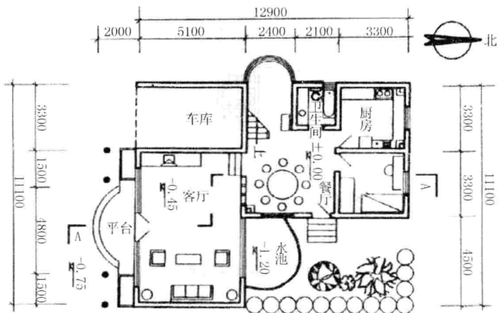
图 12 一层平面图
