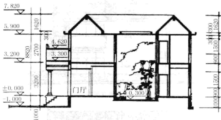
图 11 2-2 剖面图
