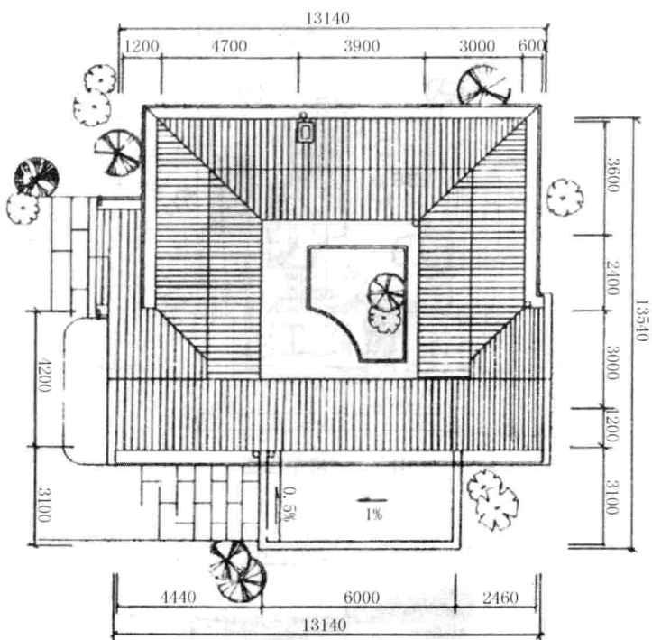
图5 屋顶平面图
