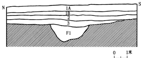
图四 T6、T7 东壁剖面图
