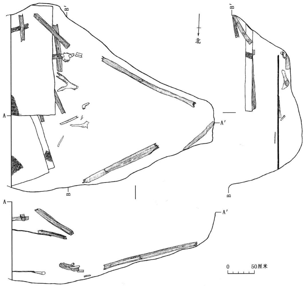
图七 F1 平、剖面图
