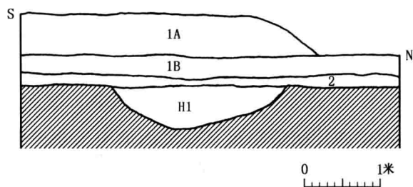
图三 T1 西壁剖面图
