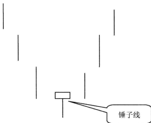
图 1—1 低位锤子线
